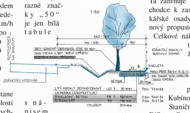
Vzorový příčný řez nového chodníku
